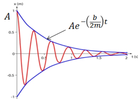
(감쇠조화진동)
