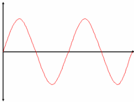
(단조화진동)
